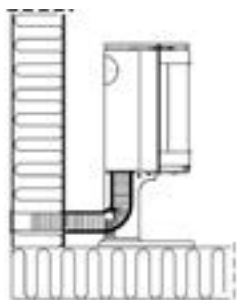
Рис. 2А, подключение сквозь внешнюю стену
