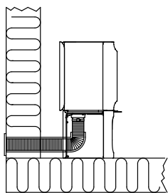
Рис. 2Б, через пол и фундаментную плиту
