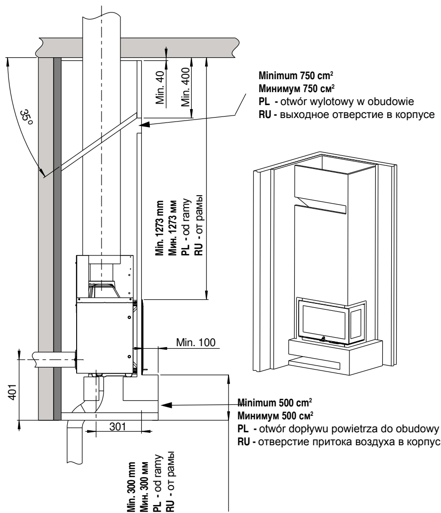
rys. 1e - przykład B / рис. 1е - пример В Jøtul I 620 F / I 620 FR / I 620 FL
