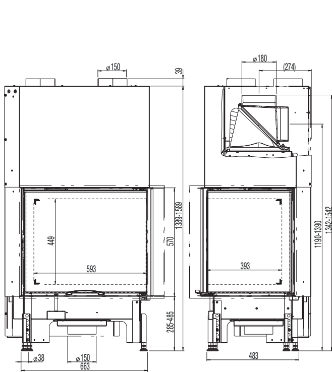
Maßstab 1:20
