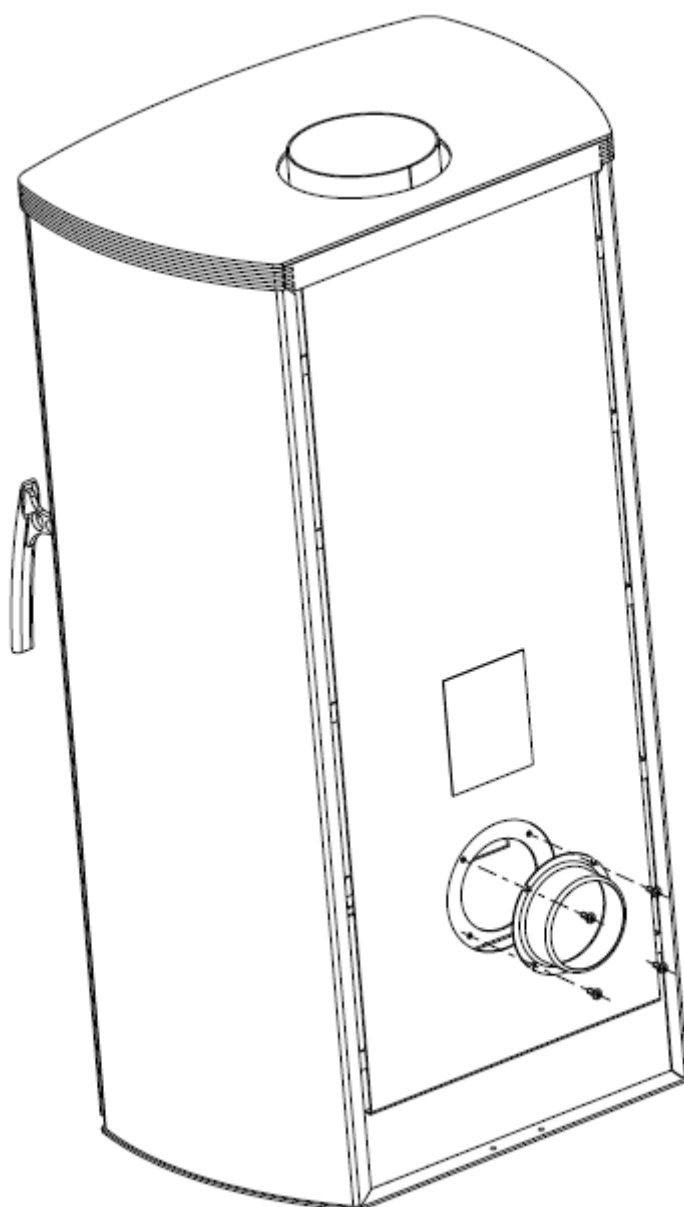
Maintaining pipe support for combustion air intake Inštalácia hrdla pre prívod spaľovacieho vzduchu Instalace hrdla pro přívod spalovacího vzduchu Az égési levegő bevezetésének előkészítése
