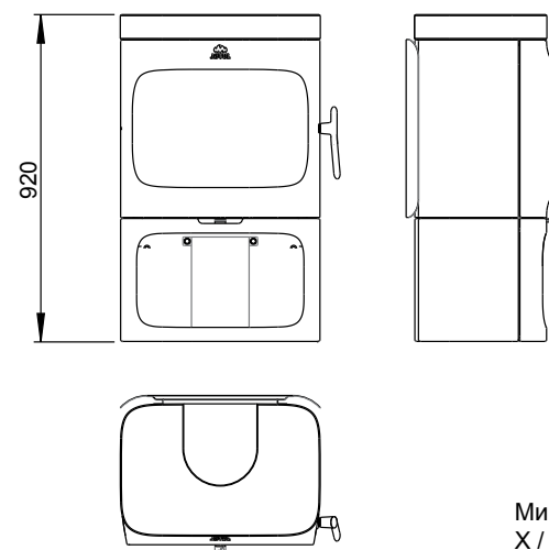
Jøtul F 305 модель на базе с верхней стеатитовой плитой
