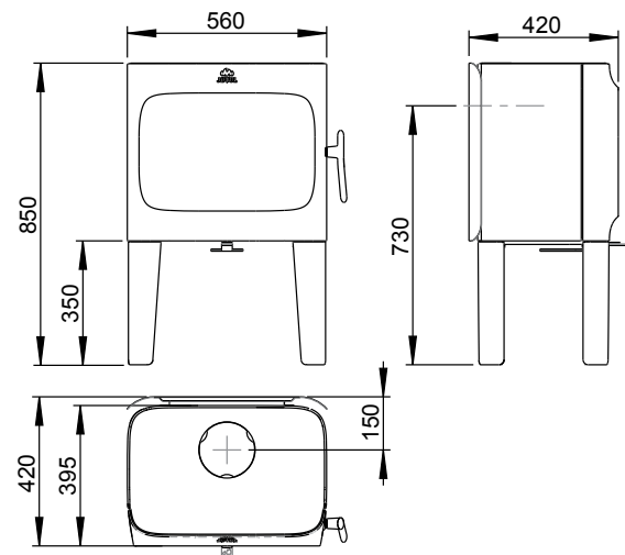
Jøtul F 305 модель на высоких ножках
