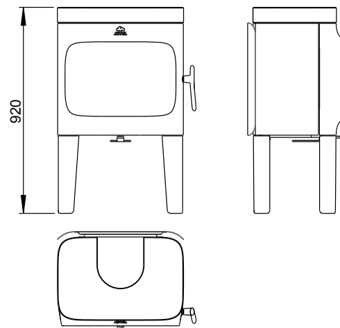
Jøtul F 305 модель на высоких ножках с верхней стеатитовой плитой
