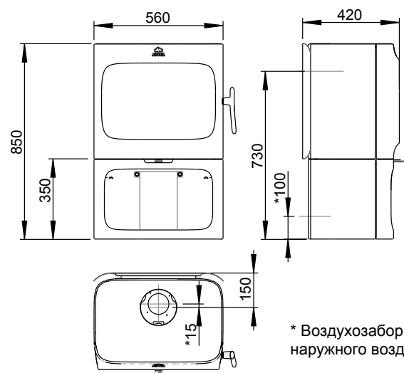
Jøtul F 305 модель на базе
