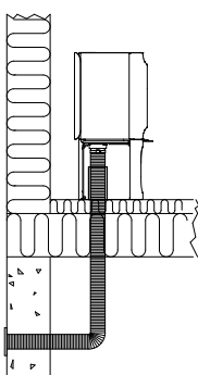
Рис. 2Г, посредственно через наружную стену
