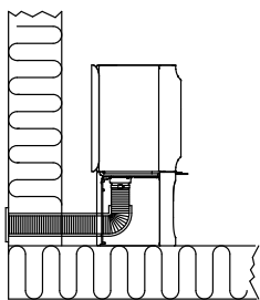
Рис. 2Б, через пол и фундаментную плиту
