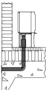
Рис. 2В, через пол и подвал
