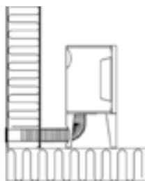
Рис. 2b, подключение через пол и фундамент
