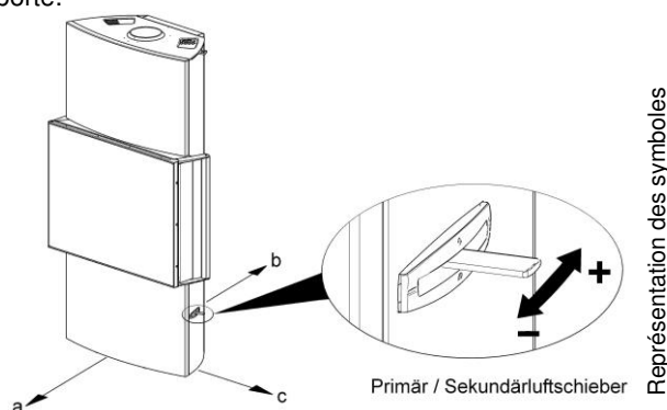
Fig. 4: régler l'arrivée d'air
