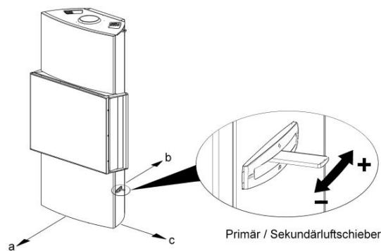
Fig. 4: Luftschieber
