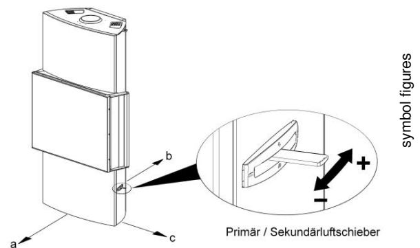
Fig. 4: air knob
